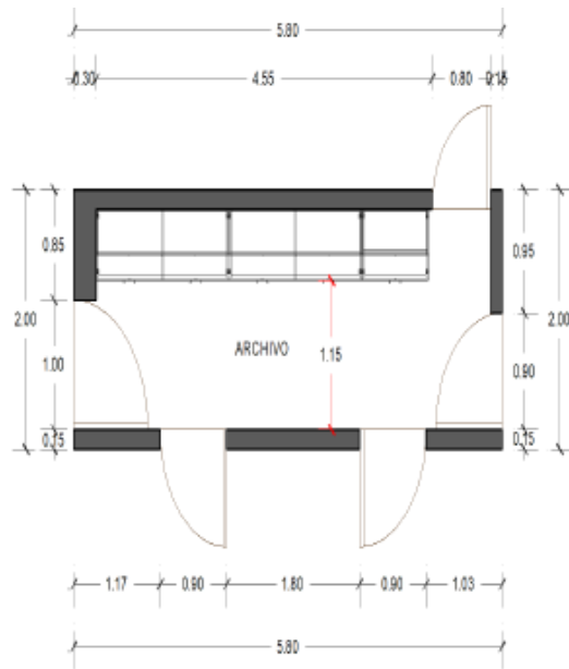
Vista en Planta
